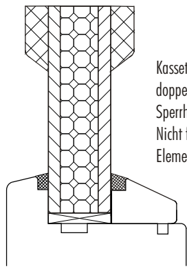
Aufdoppelung mit Nuten aus Sperrholz, bei lasierten Elementen massiv
